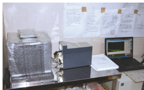
本澄寺の一室にある放射能測定所。外部の放射線が測定に影響しないように鉛の板で機材を覆っている。家賃が要らないため、検査費用は1検体500円(会員外1000円)。2か月ごとに無料測定会も行っている
